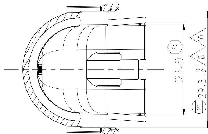
SECTION C-C Schnitt
