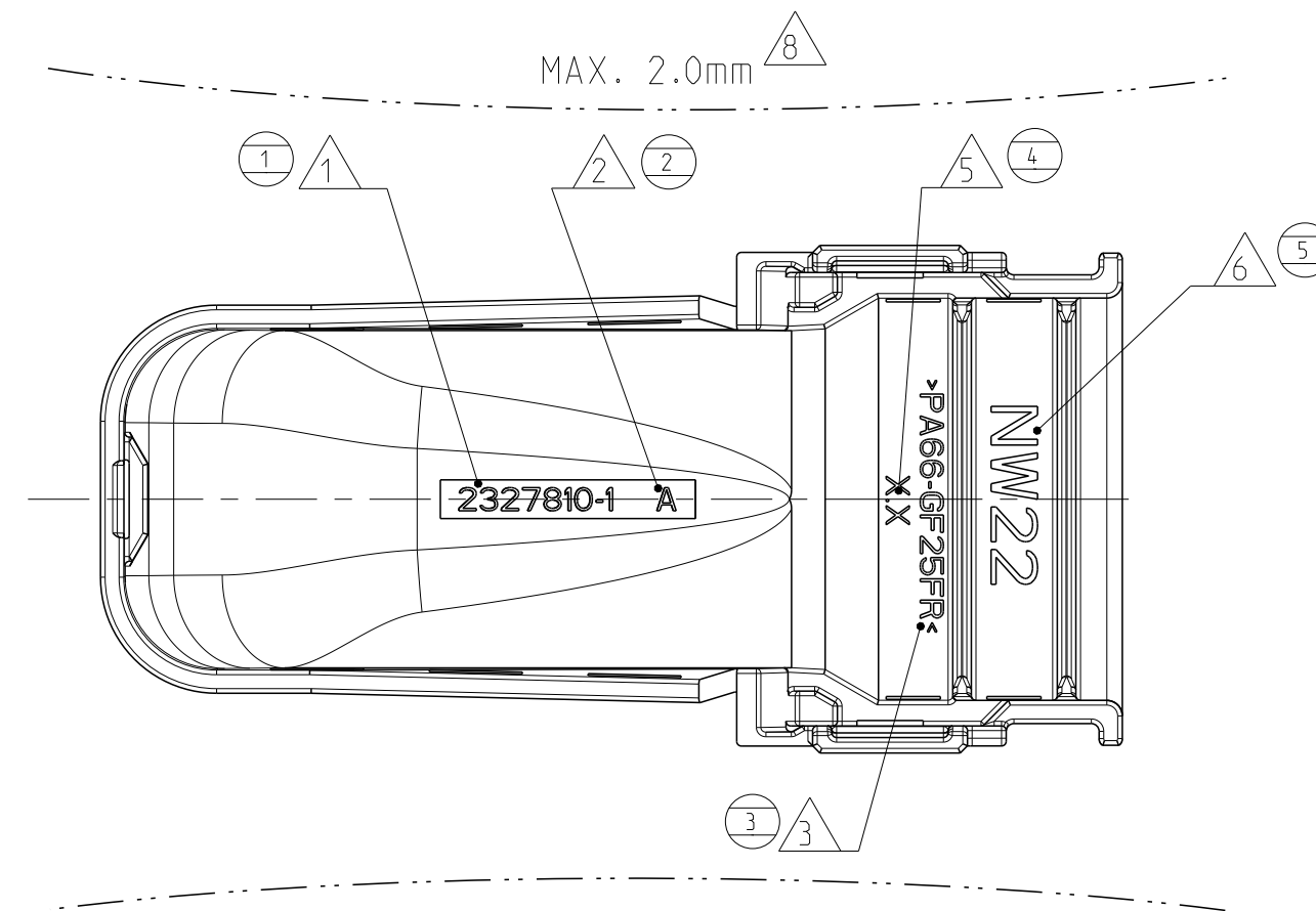
SECTION A-A Schnitt
