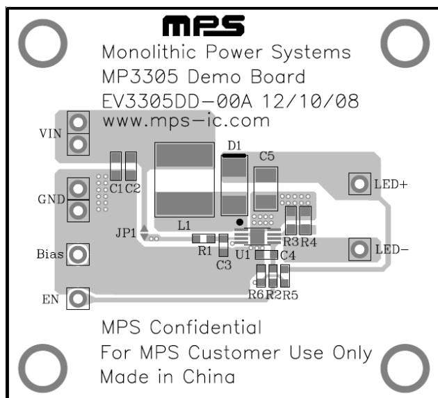
Figure 1—Top Layer
