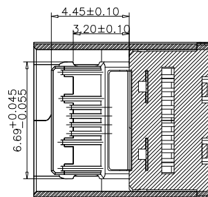
截面B-B
