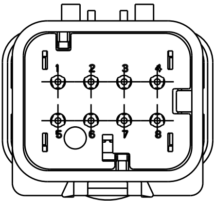
2320930-3 SCALE 2:1 KEY C
