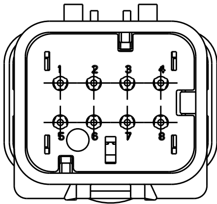
2320930-2 SCALE 2:1 KEY B
