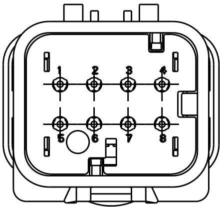
2320930-4 SCALE 2:1 KEY D
