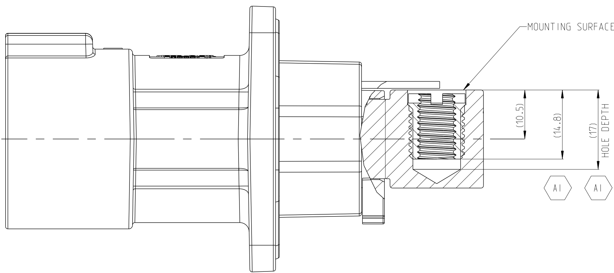
SECTION A-A
