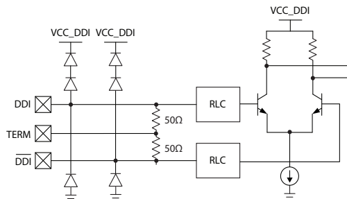
Figure 3-1: DDI0/DDI0, DDI1/DDI1
