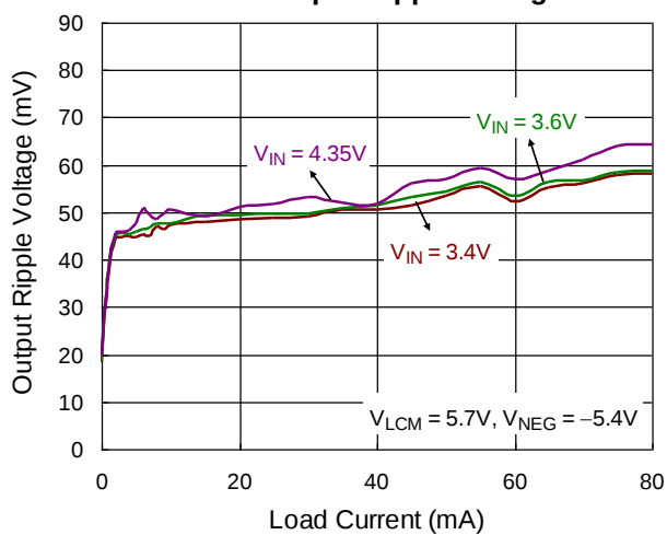
NEG Output Ripple Voltage
