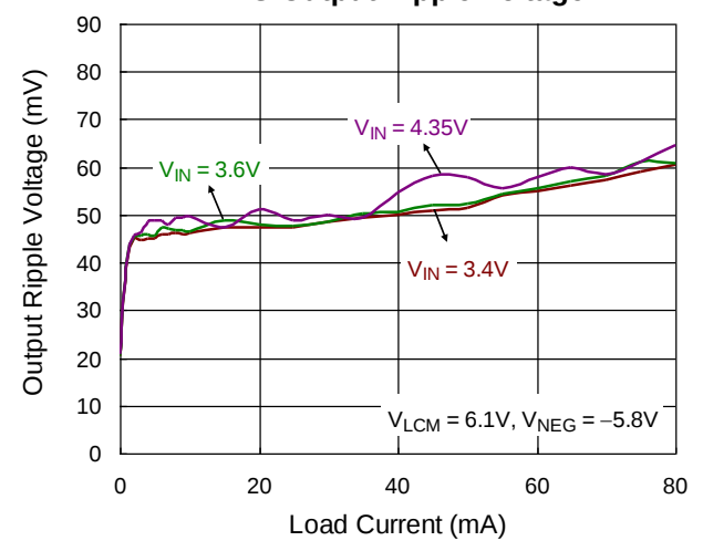
NEG Output Ripple Voltage
