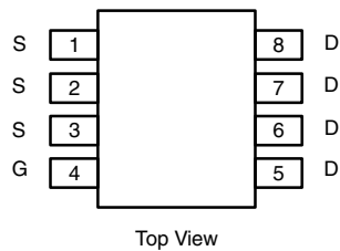
SO-8
