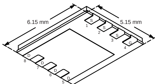
DFN8(5*6)
