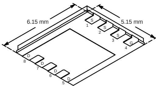
DFN8(5*6)
