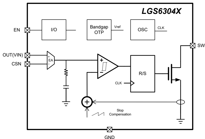
图 5 内部功能框图
