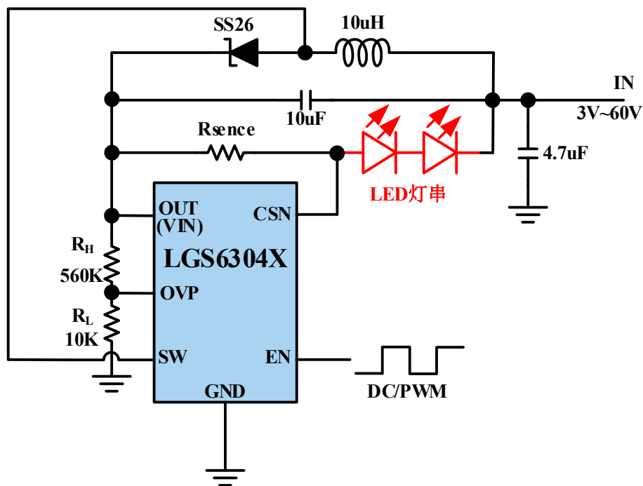
图 3.c LGS6304X 升/降压模式典型应用拓扑( V_{IN} < V_{LED} 或 V_{IN} > V_{LED} )
