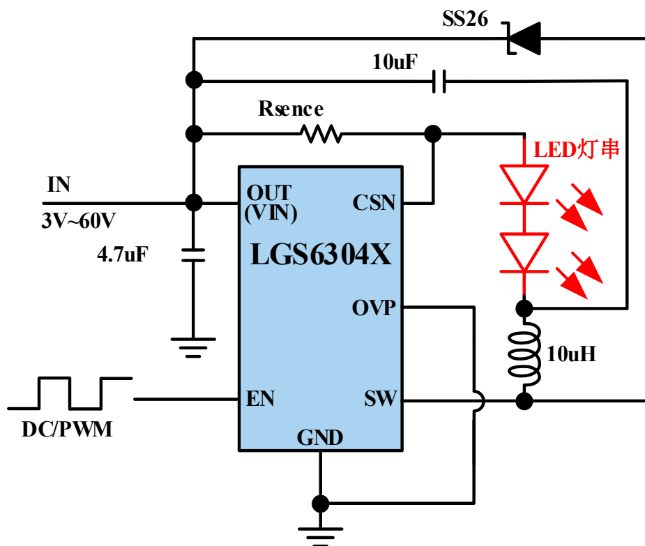
图 3.a LGS6304X 降压模式典型应用拓扑( V_{IN} > V_{LED} )
