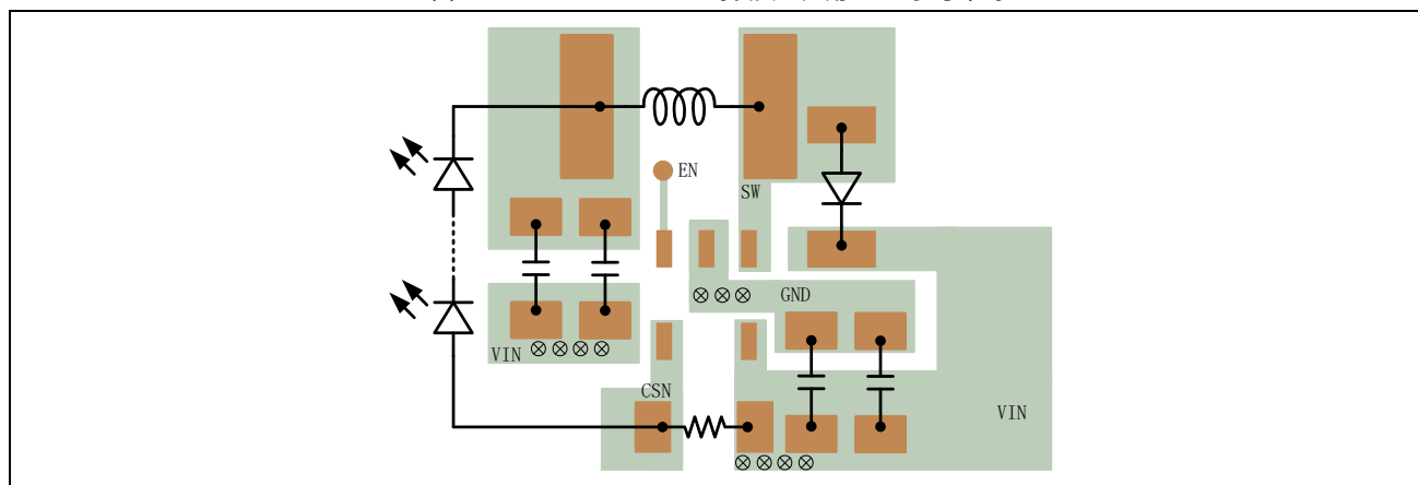
图 15.2 BUCK 型 SOT23-5 封装典型应用 PCB 参考布局
