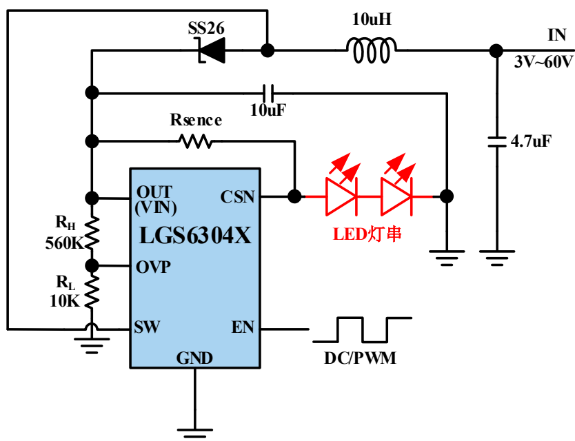
图 3.b LGS6304X 升压模式典型应用拓扑( V_{IN} < V_{LED} )
