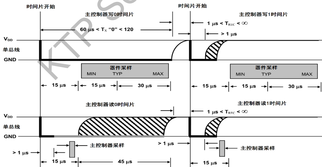
图 2-12 读/写时隙时序图
