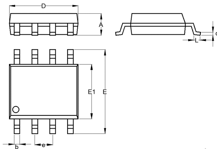
SOP8 外形图
