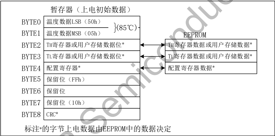
图 2-5 DS18B20 存储器映射
