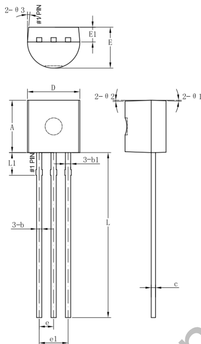
T0-92 外形图
