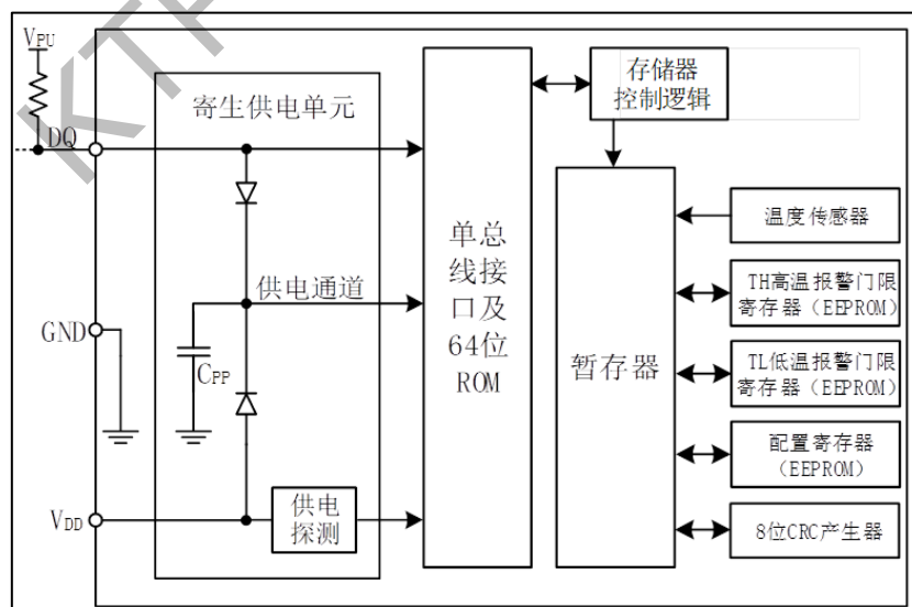
图 2-1 产品功能框图
