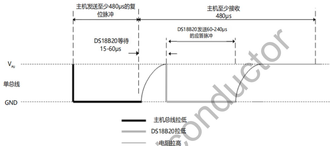
图 2-11 初始化序列时序
