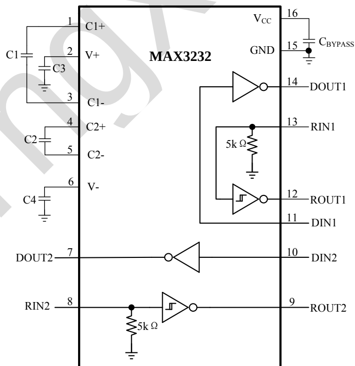
MAX3232 典型应用图
