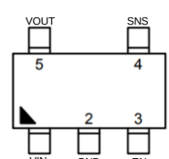
SOT-23-5
