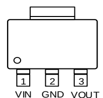
SOT-89-3 ( R-Type )
