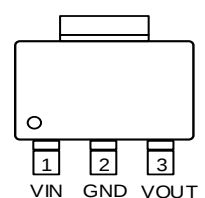
SOT-89-3 ( R-Type )
