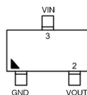
SOT-89-3 ( L-Type )
