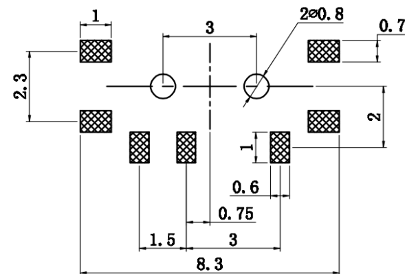
安装参考图
