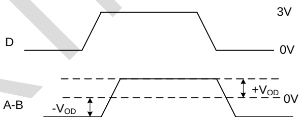
图2 驱动器数据传输速率测试
