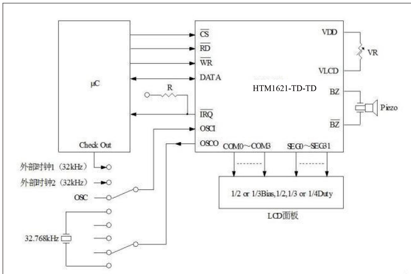
参考应用线路图
