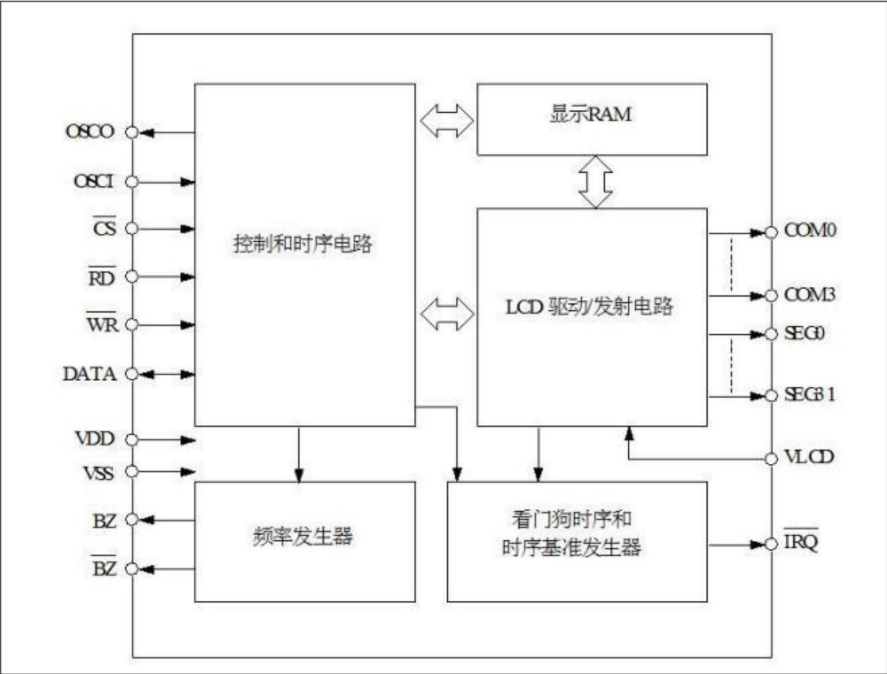
功能框图
