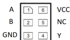
DFN1510-6
