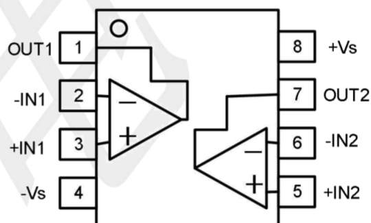
SOP8
