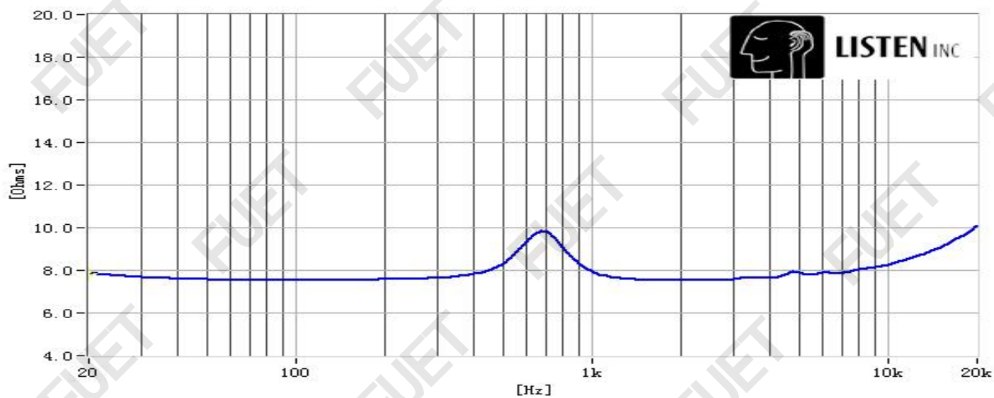
阻抗曲线
