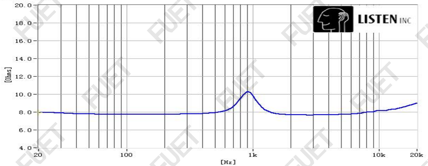
阻抗曲线
