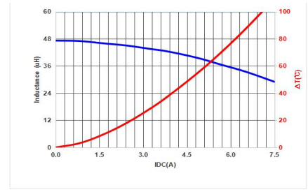
MMPC1005-470MT
