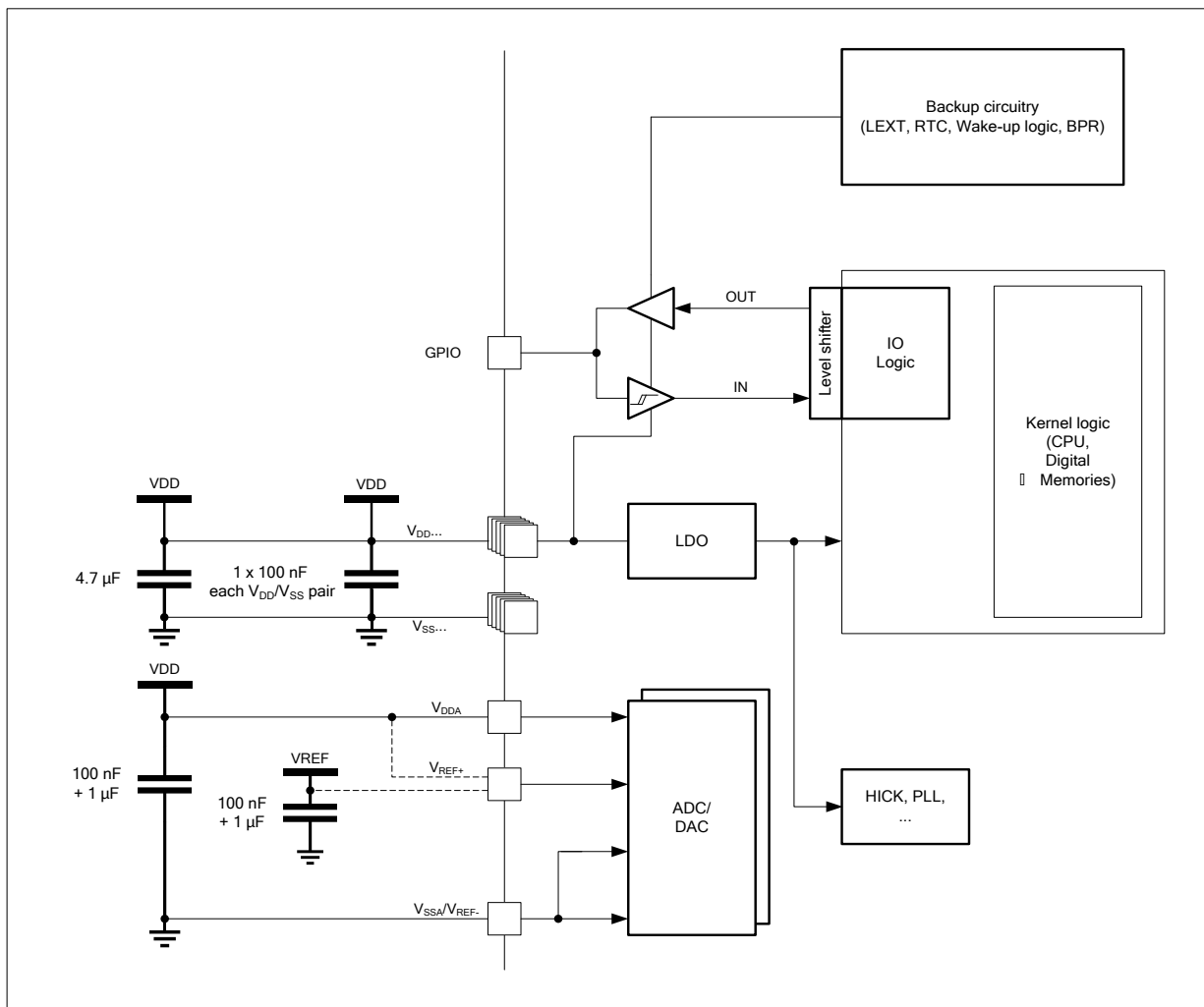
图 7. 供电方案
