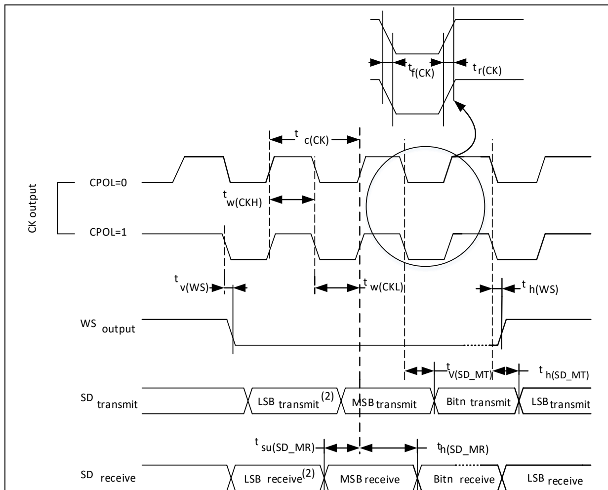
图 26. I 2 S 主模式时序图 (Philips 协议)
