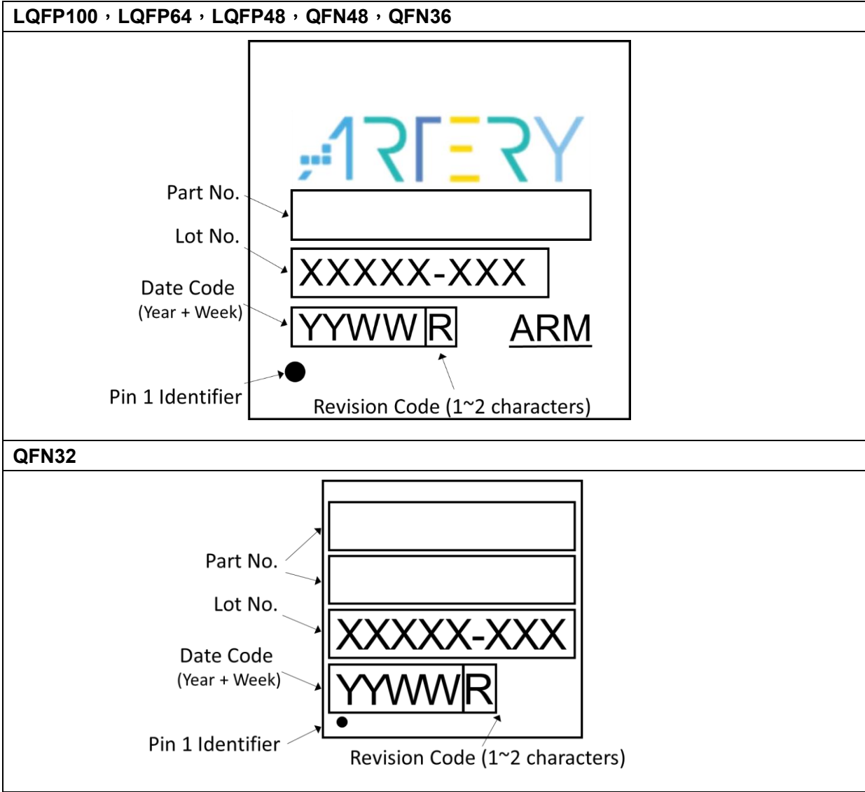
图 40. 丝印示意图
