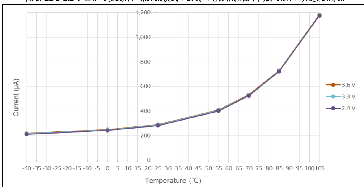
图 10. LDO 在额外低功耗模式时, 深睡眠模式下的典型电流消耗在不同的 V DD 时与温度的对比
