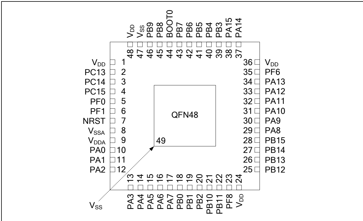
图 4. AT32F423 系列 QFN48 引脚分布
