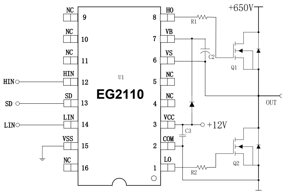
图 6-1. EG2110 典型应用电路图
