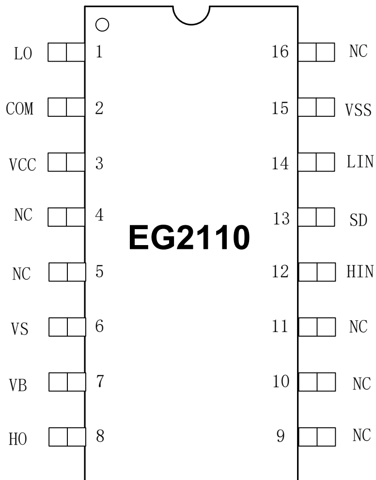
图 4-1. EG2110 管脚定义
