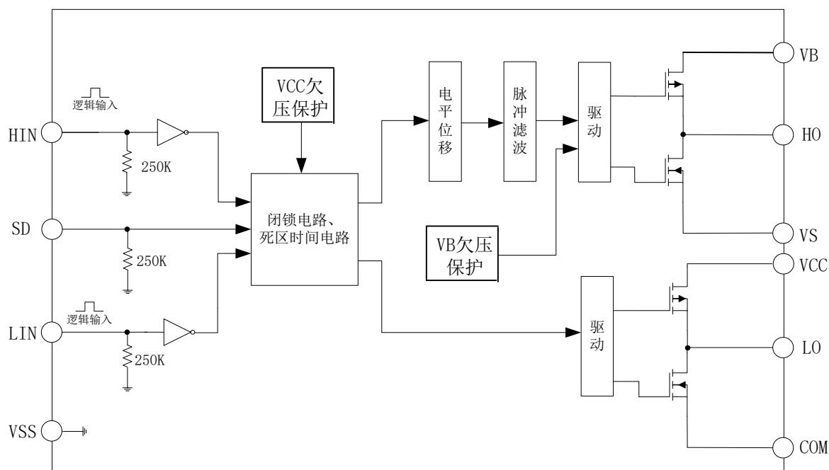
图 5-1. EG2110 内部电路图
