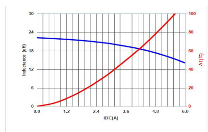
MMPC1003-220MT
