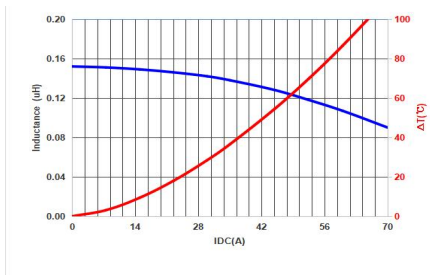
MMPC1003-R47MT
