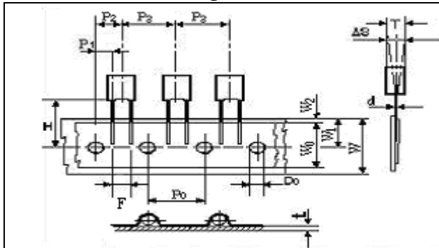
Fig.1 P=5.0/7.5mm
