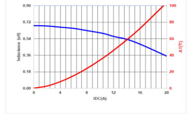
MMPC0602-2R2MT
