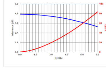
MMPC0602-8R2MT
