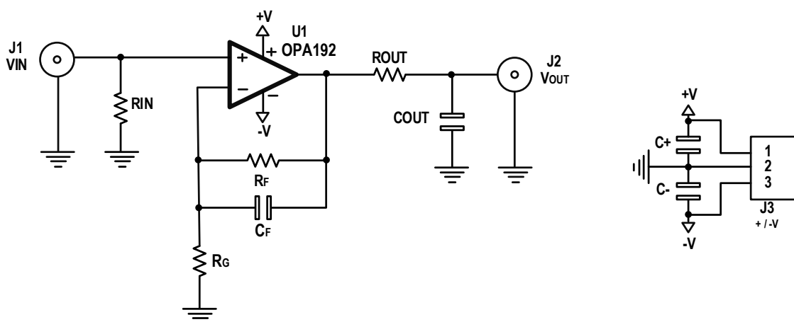
图39. 同相配置的运算放大器原理图
