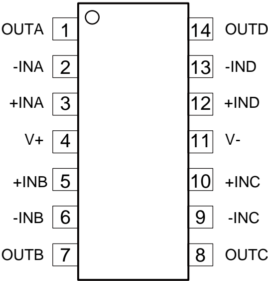
OPA4177ARZ 引脚配置 (俯视图) SOIC-14 封装和 TSSOP-14 封装
