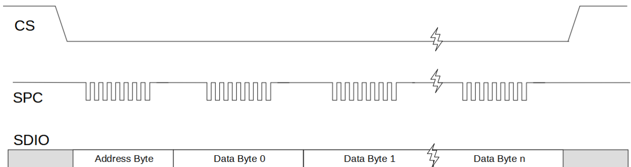
SPI : Mode 3
