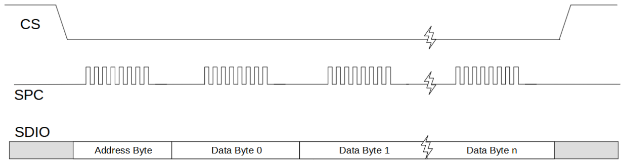
SPI : Mode 0
