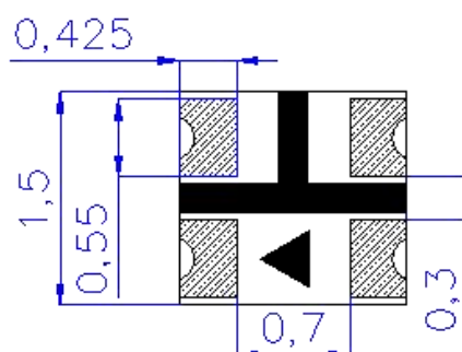
建议焊盘 仅供参考
