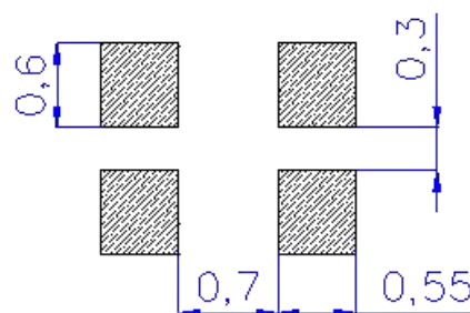
建议焊盘 仅供参考
