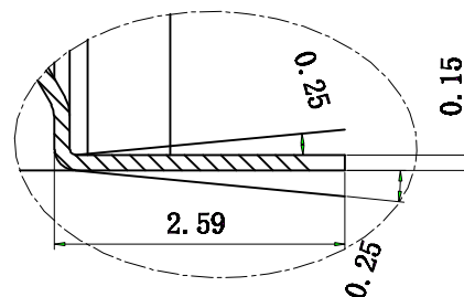
DETAIL B Sec:6:1
