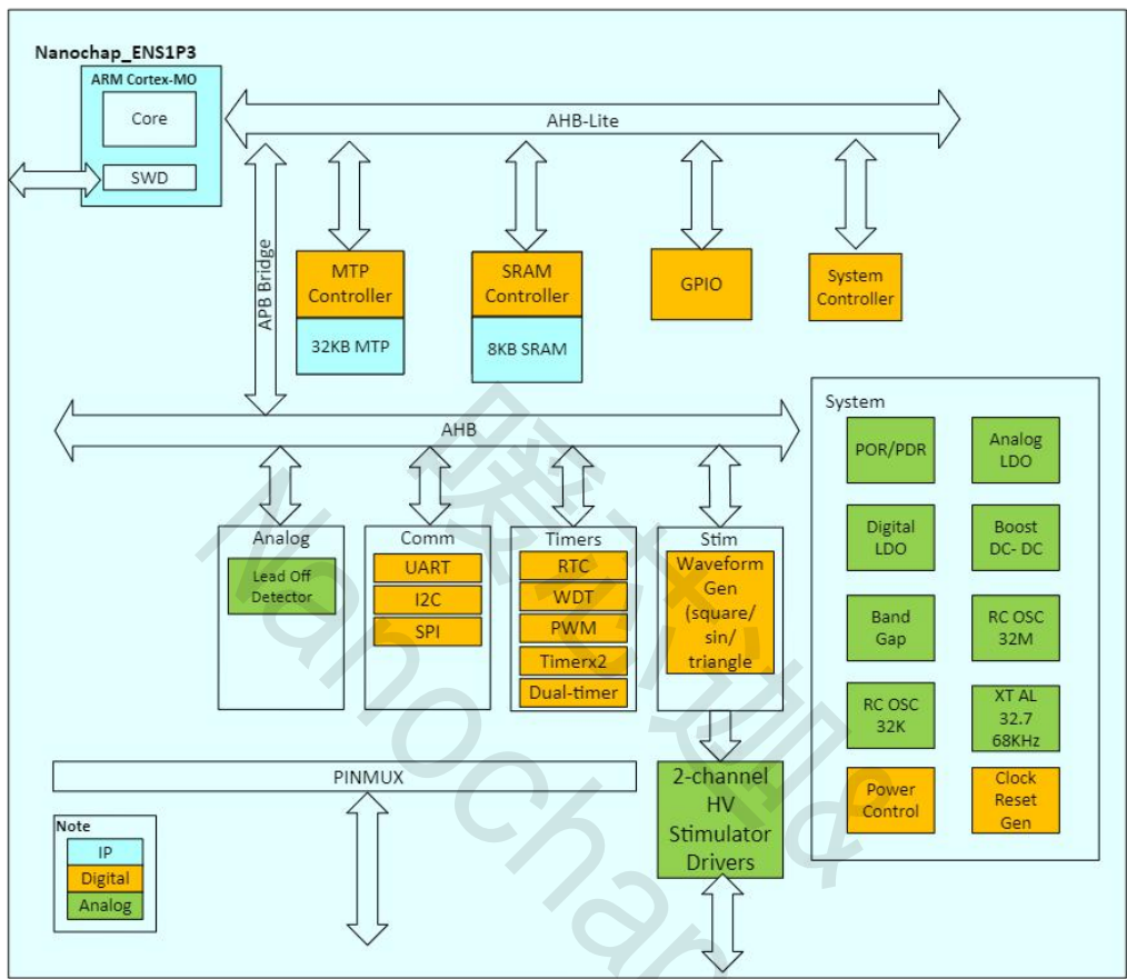
图 6 NNC6121EVKB 芯片框图
