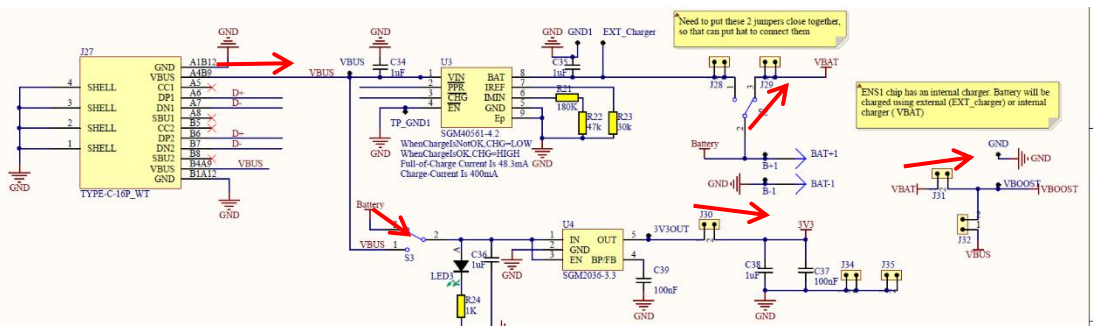
图 11 锂电池供电
