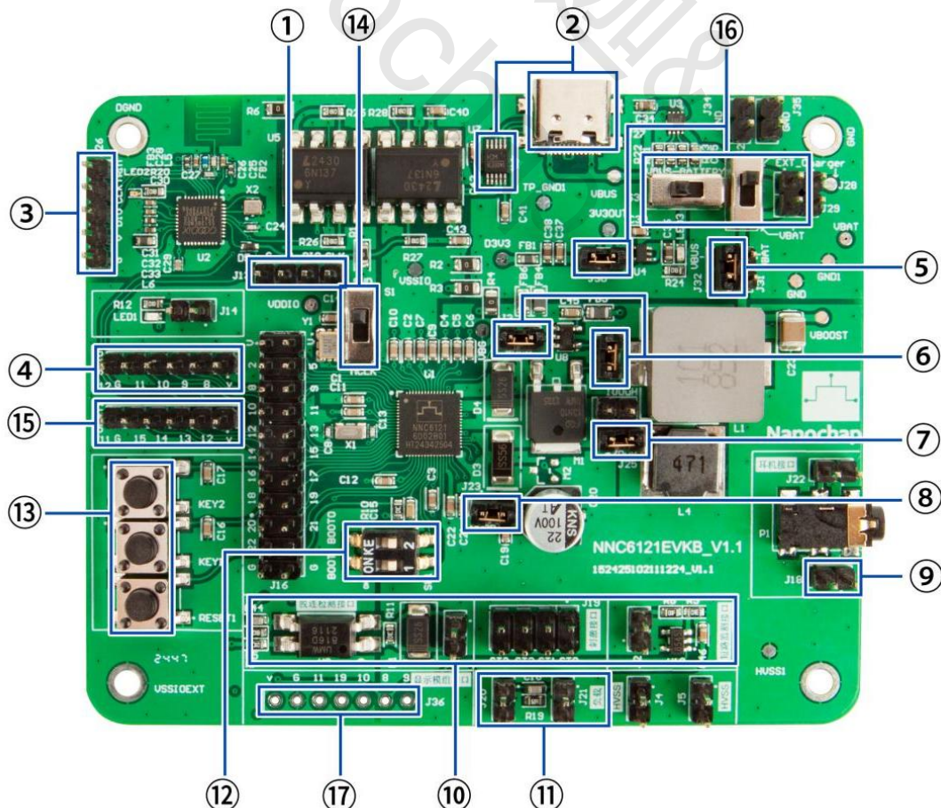
图 1 NNC6121EVKB 双通道开发板图
