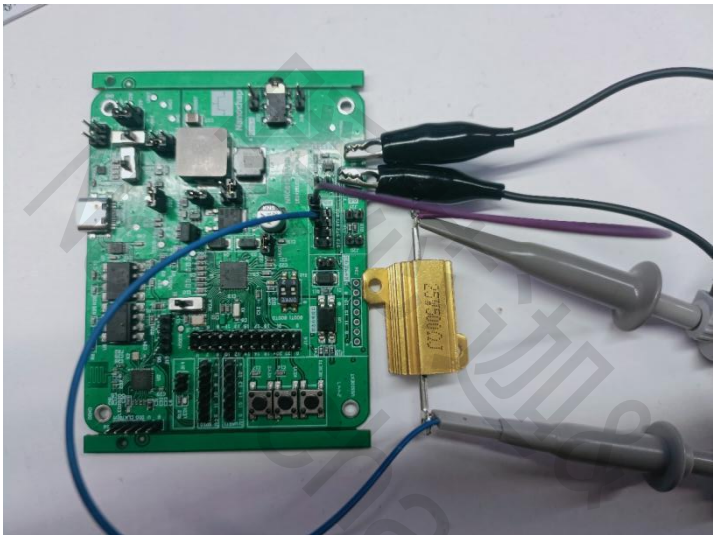
图 19 示波器探头连接方法
