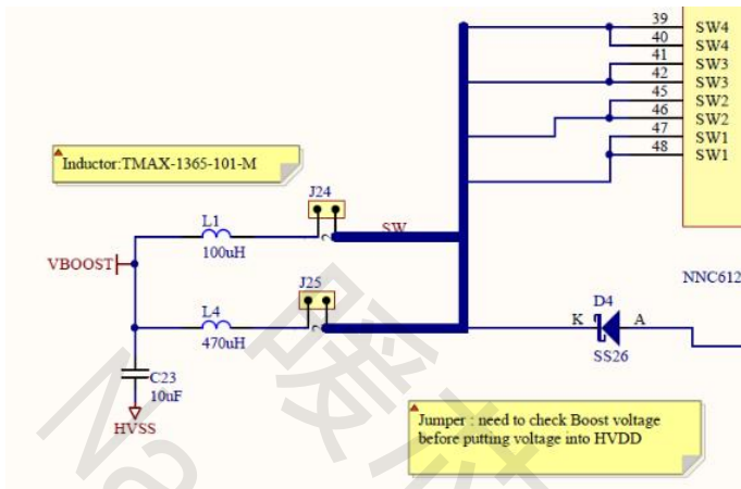
图 2 电感、电容、肖特基二极管位置
