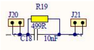
图 14 NNC6121EVKB 刺激电流输出位置及板上负载
