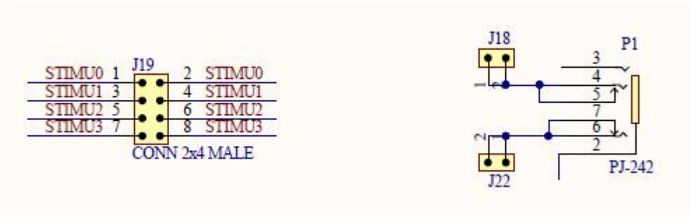
图 14 NNC6121EVKB 刺激电流输出位置及板上负载
