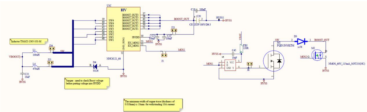
图 8 NNC6121EVKB 的 BOOST 电路
