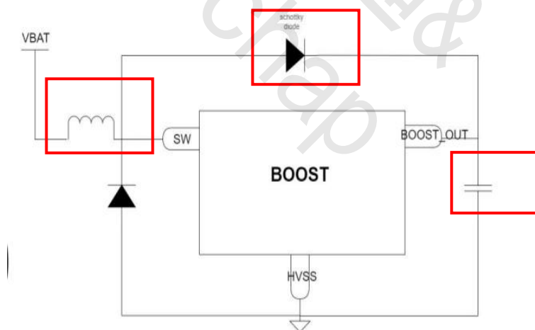
图 7 NNC6121EVKB 的 BOOST 电路
