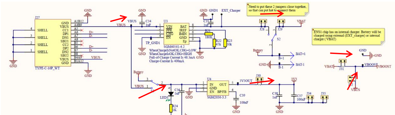
图 10 Type-C 接口输入供电图示
