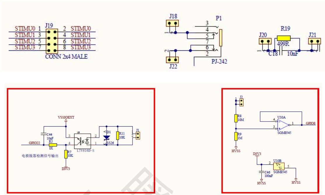
图 4 电刺激输出接口及板上测试电路
