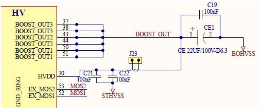
图 3 J23 跳帽原理图位置
