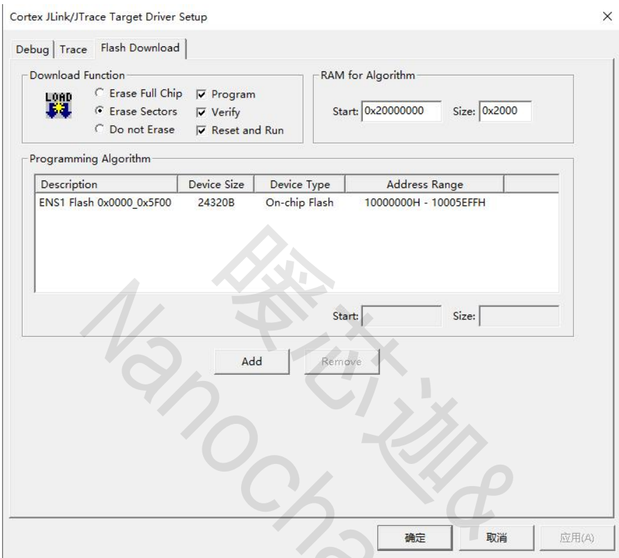
图 16 KEIL 的 flash 烧录文件选择界面
