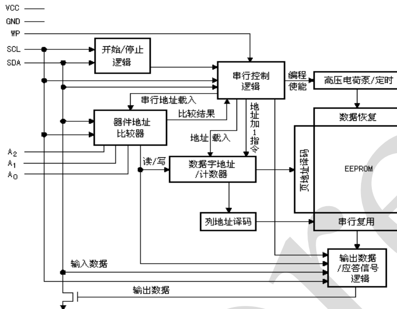
图 1、功能框图
