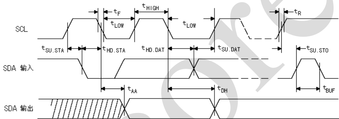
图 5、总线时序
