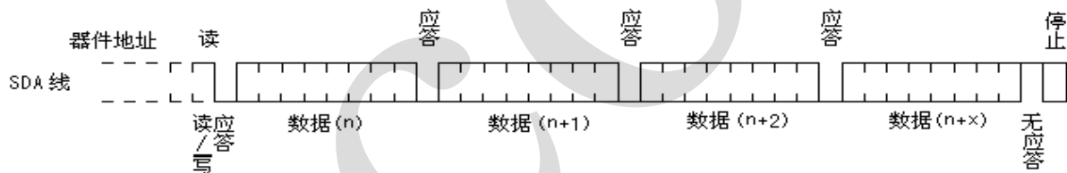
图 12、顺序地址读操作
