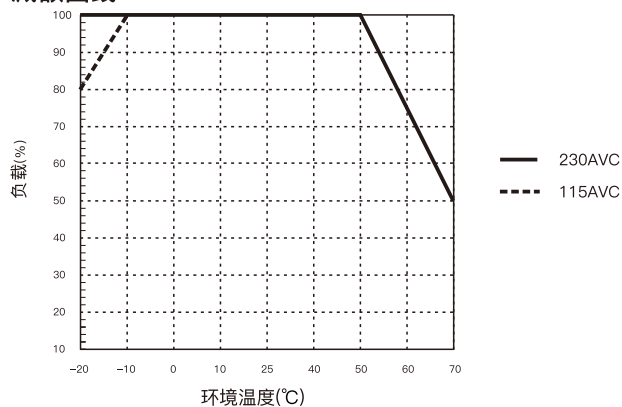
减额曲线
