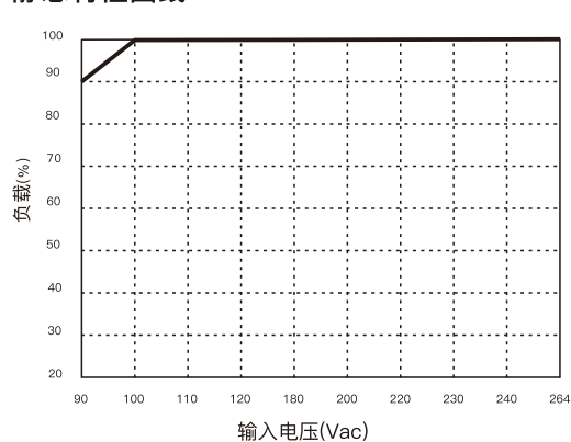
静态特性曲线
