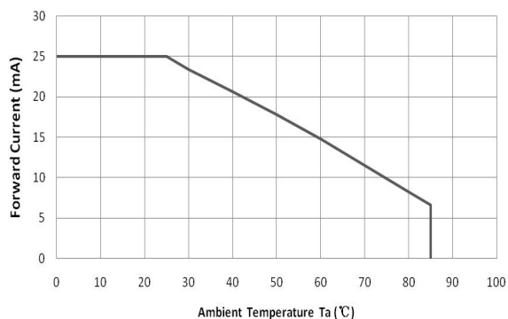
最大正向电流与环境温度特性曲线
