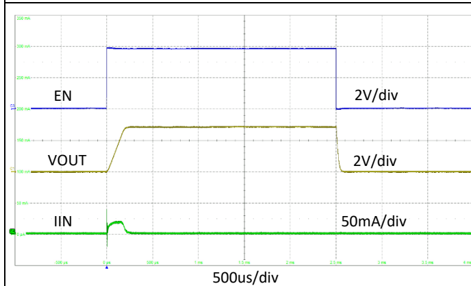
Fig 9. EN 启动、关闭
