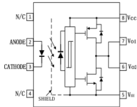
DIP8-M
