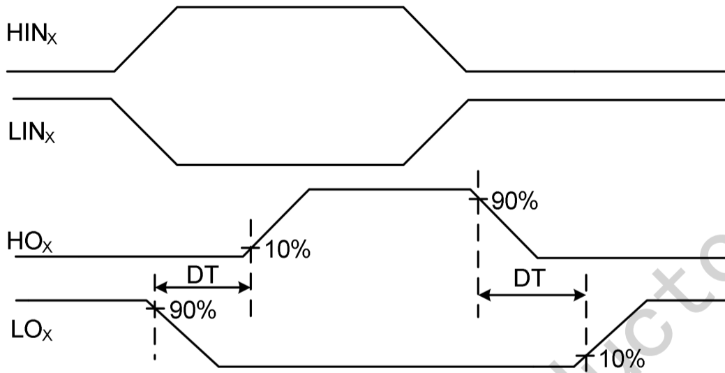
图 6-3 死区时间波形定义
