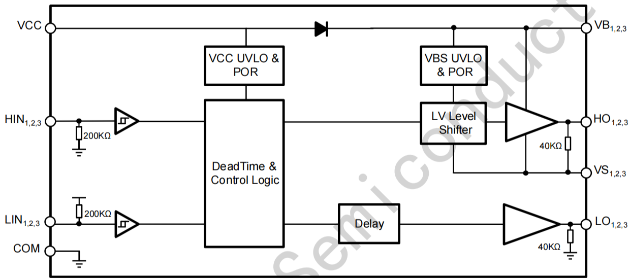
图 7-1 SD6288功能框图
