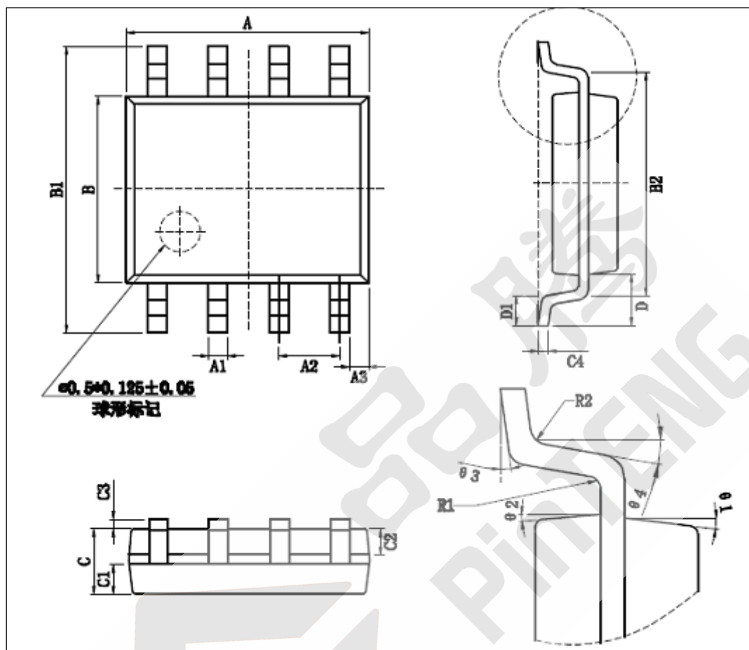
图 6 SOP8 封装
