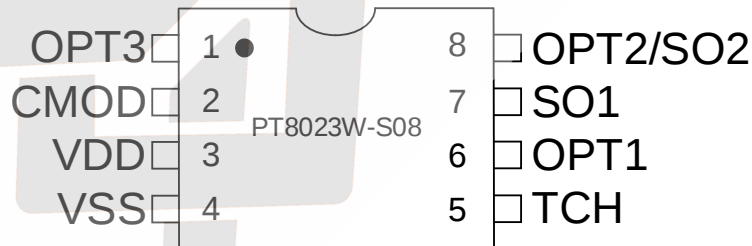
图 1 SOP8 管脚示意
