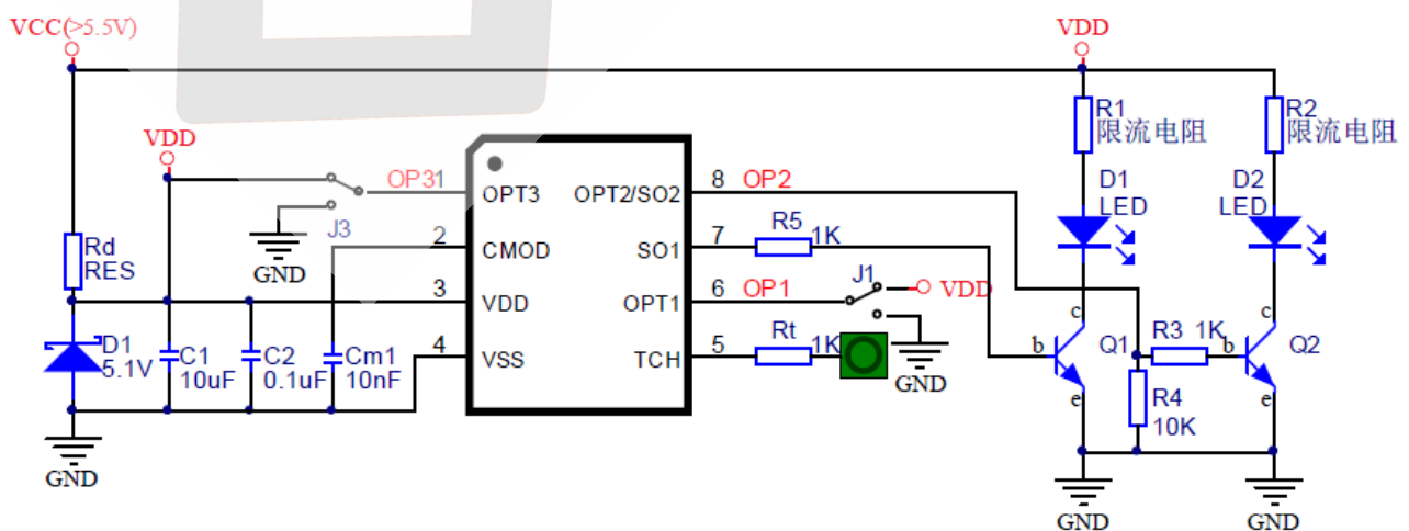
图 5 单输入双输出直流高压供电应用电路
