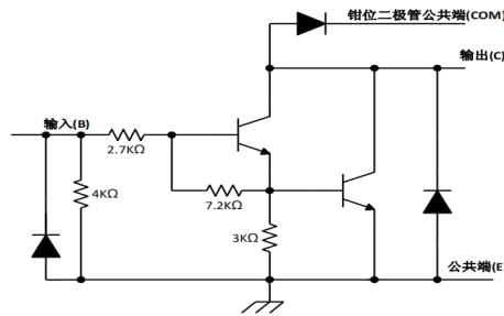
ULN2002 单路达林顿驱动电路原理图
