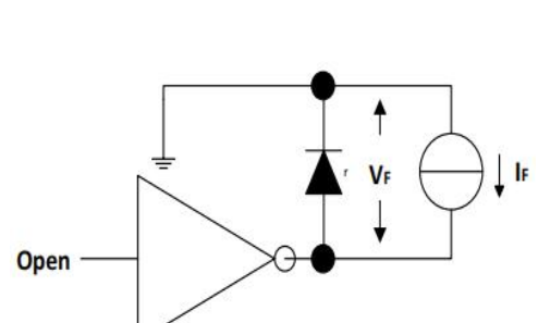
图 6 V F 测试电路
