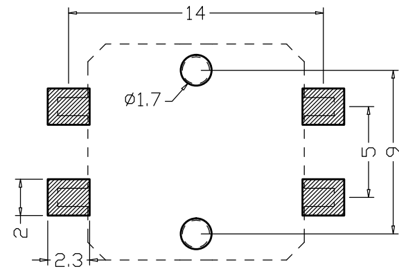
PCB线路板图
