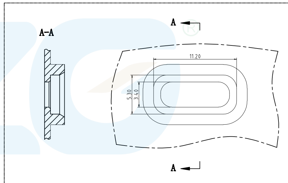
外壳参考设计图
