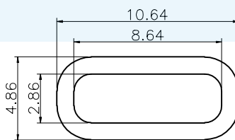
建议胶圈尺寸
