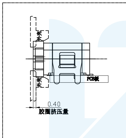
组装示意图
