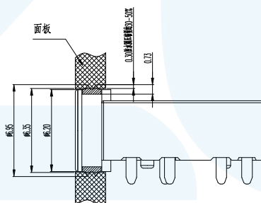
面板开孔建议尺寸(ø6.35)
