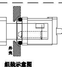
组装示意图
