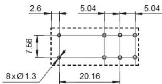
安装尺寸 (底视图)
