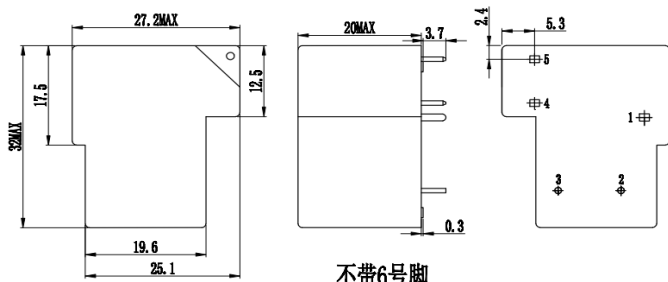
不带6号脚
