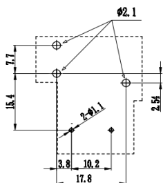
不带6号脚
