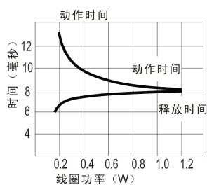
性能曲线图
