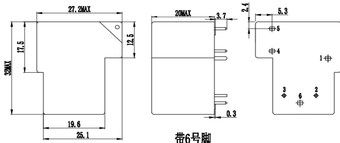
外形图
