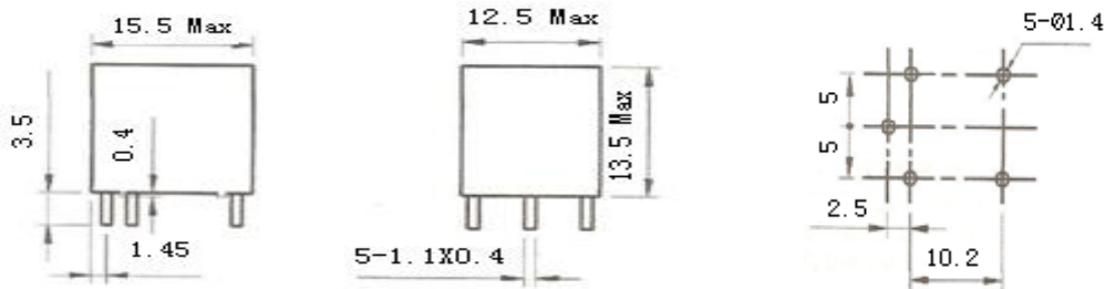
外形尺寸图
