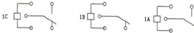
接线图 (底视图)
