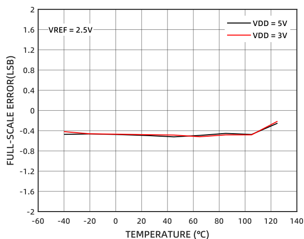
图 15 满量程误差的温度特性
