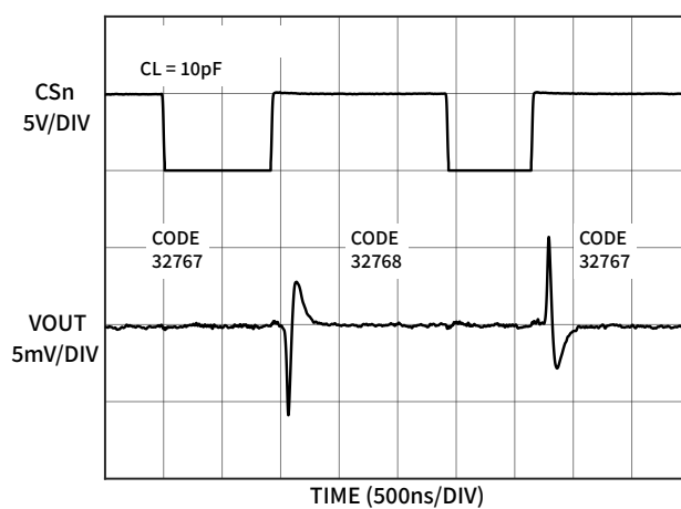
图 17 主进位翻转毛刺脉冲
