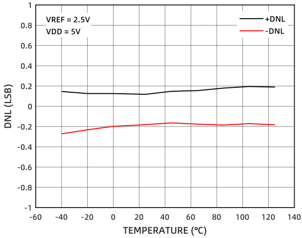
图 8 DNL 的温度特性 (5V)
