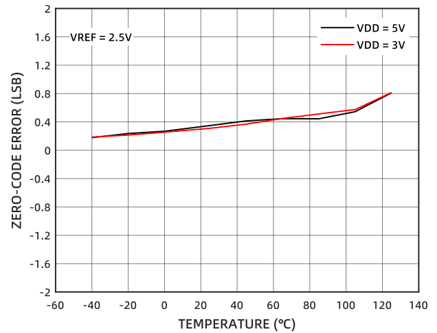
图 13 零码输入误差的温度特性
