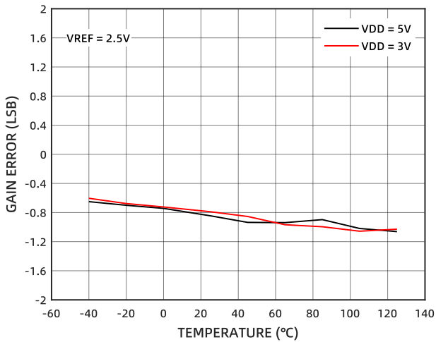
图 12 增益误差的温度特性
