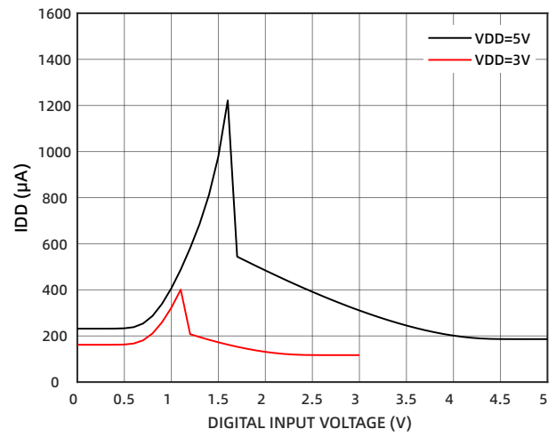
图 11 IDD 随输入电压的变化
