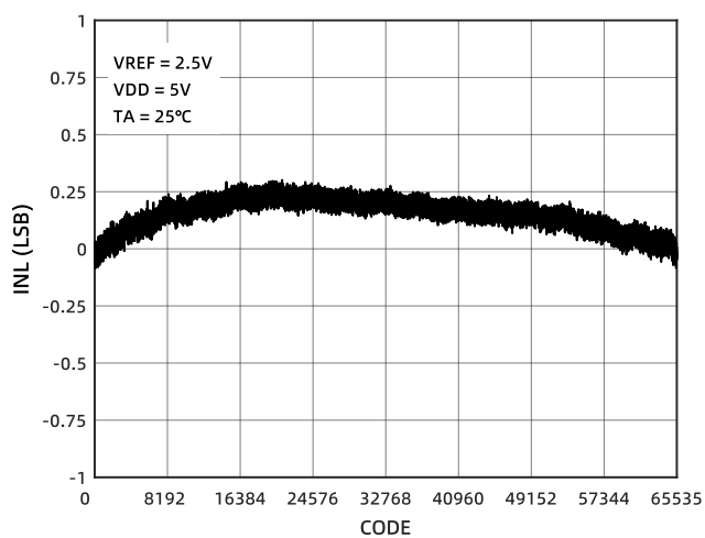
图 2 INL
