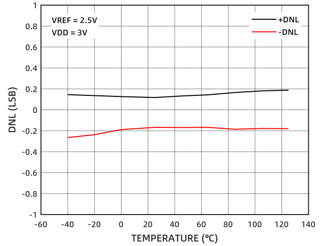
图 9 DNL 的温度特性 (3V)
