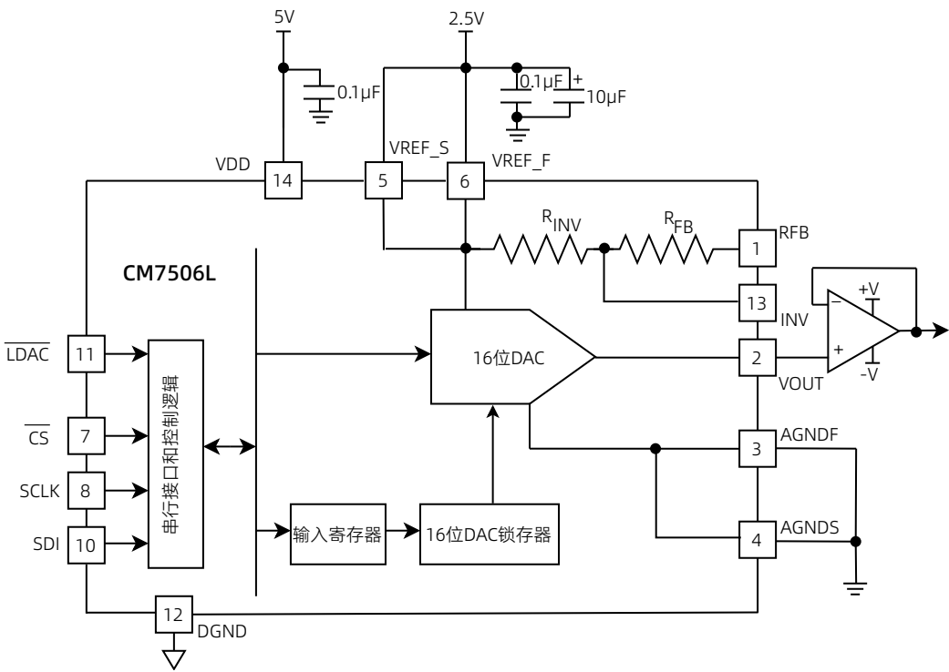
图 20 典型连接
