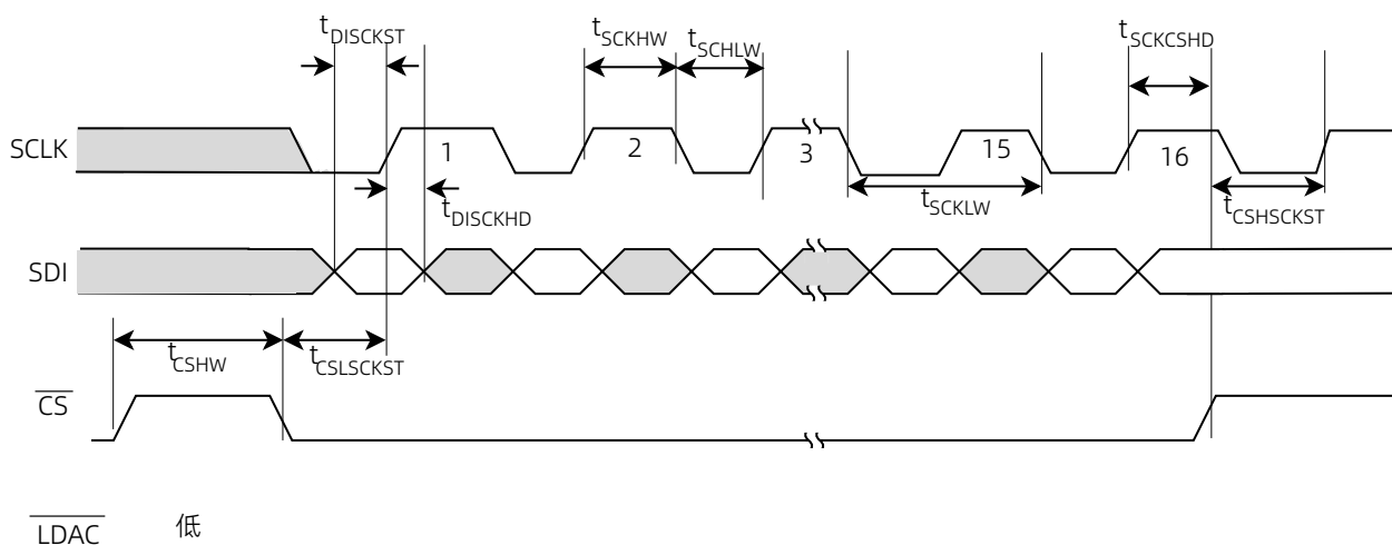
图 1 SPI 时序图
