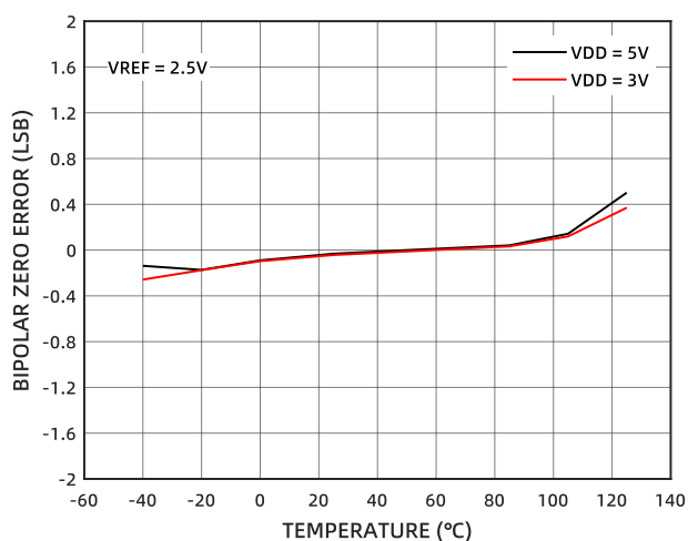
图 14 双极性零压失调误差的温度特性
