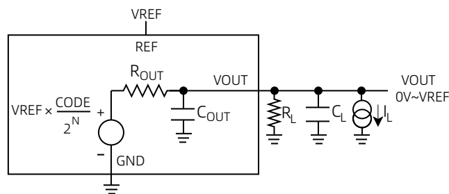
图 18 VOUT 管脚等效电路
