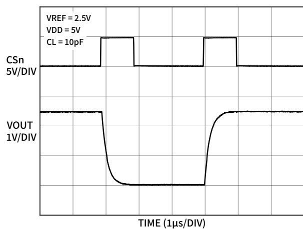
图 16 满量程高低电平转换
