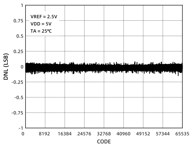
图 6 DNL
