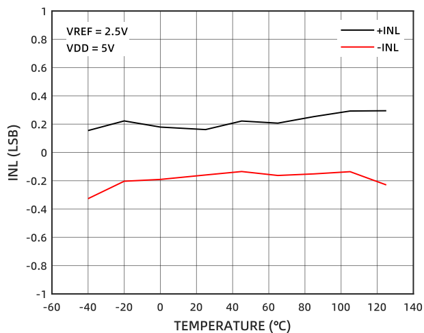
图 4 INL 的温度特性 (5V)
