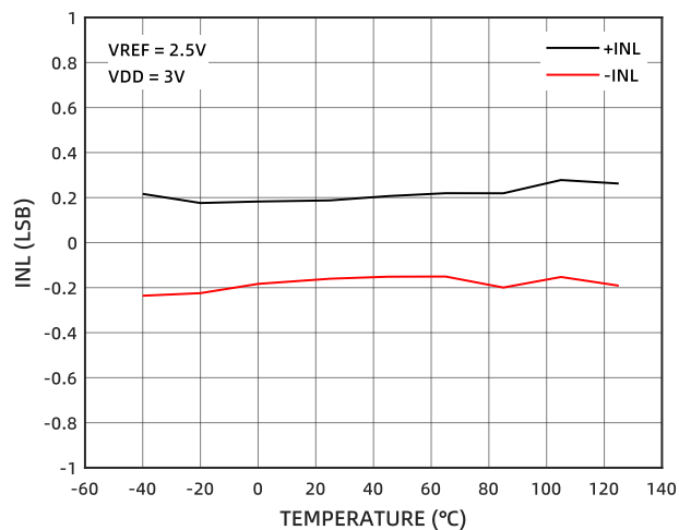
图 5 INL 的温度特性 (3V)
