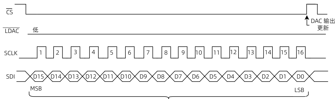
图 19 时序图
